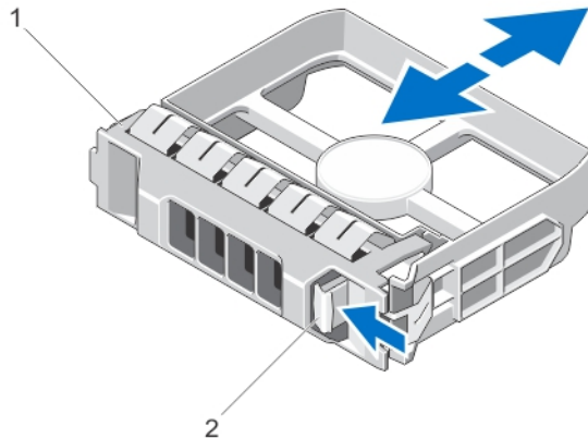
그림 19. 3.5인치 하드 드라이브 보호물 분리 및 설치
