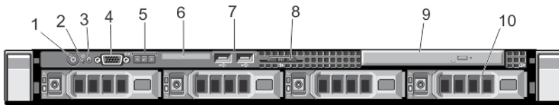
그림 1. 전면 패널 구조 및 표시등—3.5인치 하드 드라이브 4개를 포함하는 시스템
