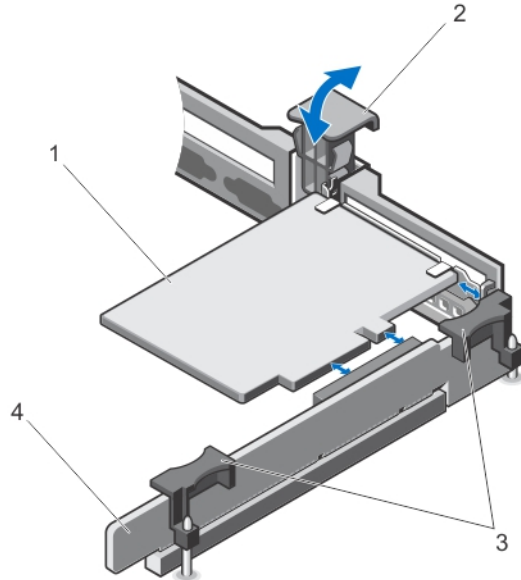
그림 30. 확장 카드 라이저 1에서의 확장 카드 분리 및 설치
