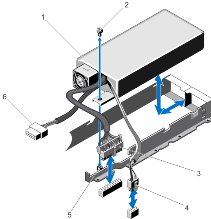
그림 41. 비중복 전원 공급 장치 분리 및 설치
