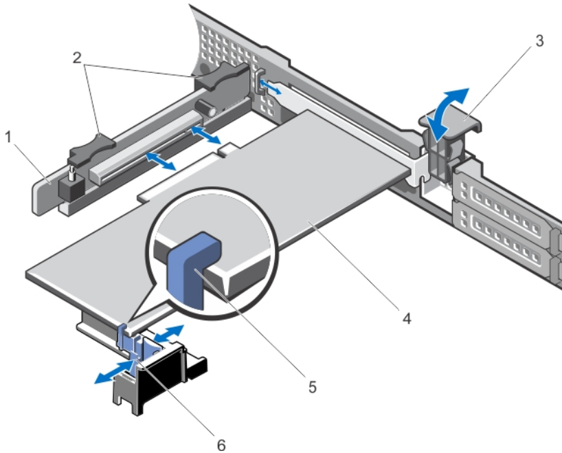
그림 31. 확장 카드 라이저 2에서의 확장 카드 분리 및 설치
