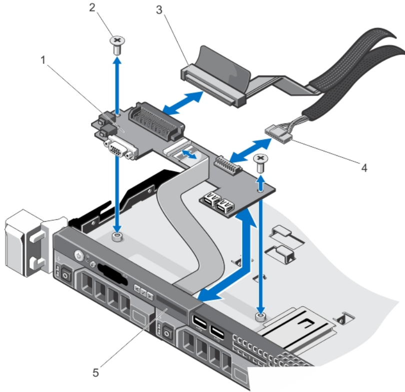
그림 55. 제어판 모듈 분리 및 설치—핫 플러그 가능 3.5인치 하드 드라이브 시스템
