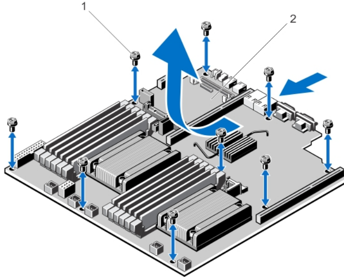
그림 60. 시스템 보드 분리 및 설치
