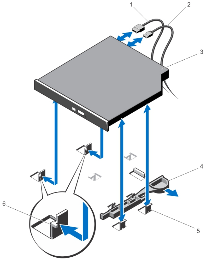
그림 27. 광학 드라이브 분리 및 설치(케이블 연결된 하드 드라이브 시스템)
