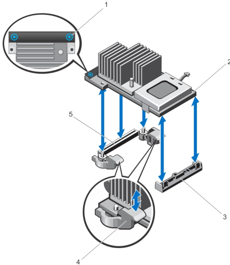
그림 37. 내장형 저장소 컨트롤러 카드 분리 및 설치
