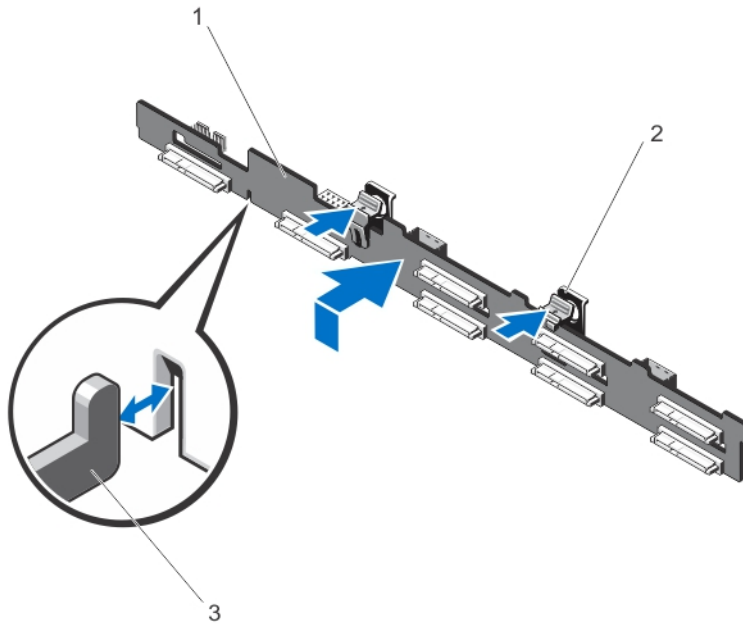
그림 50. 8개 하드 드라이브 후면판 분리 및 설치
