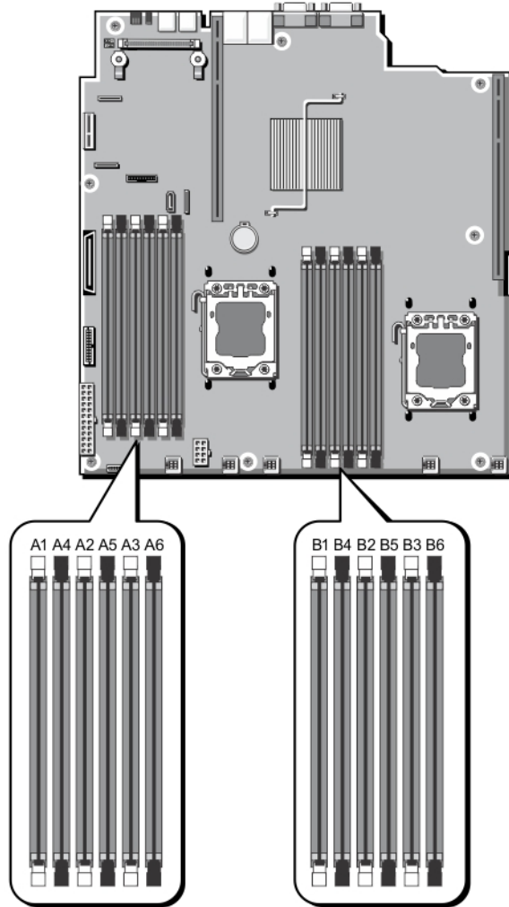
그림 14. 메모리 소켓 위치
