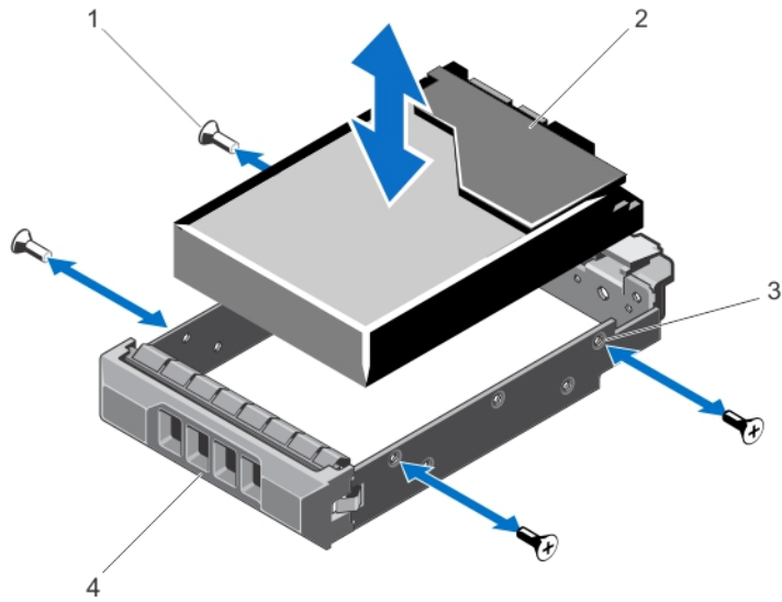
그림 25. 하드 드라이브 캐리어에서 케이블 연결된 하드 드라이브 분리 및 설치
