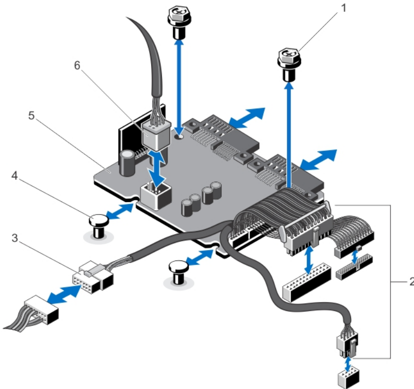
그림 59. 배전 보드 분리 및 설치
