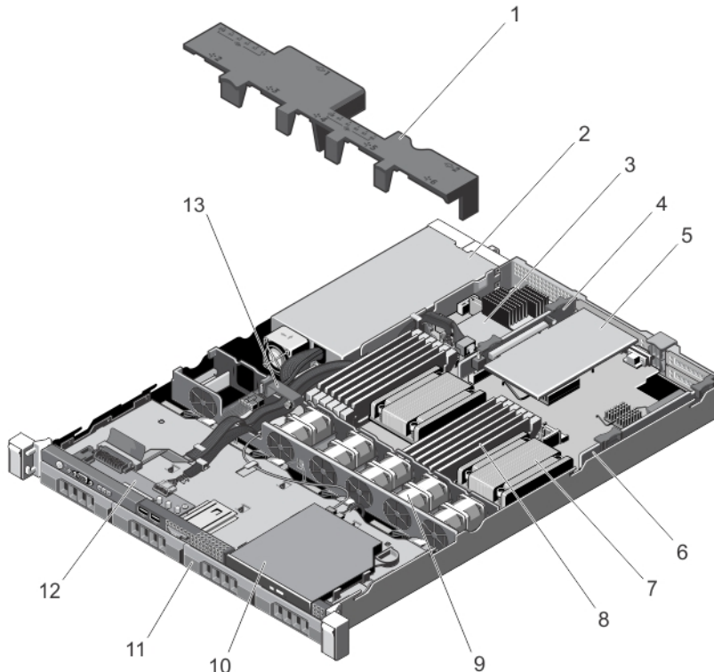
그림 11. 시스템 내부—비중복 전원 공급 장치 포함
