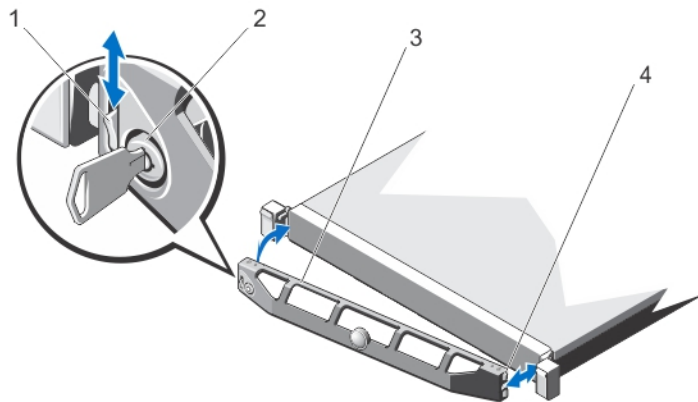
그림 9. 전면 베젤 설치 및 분리
