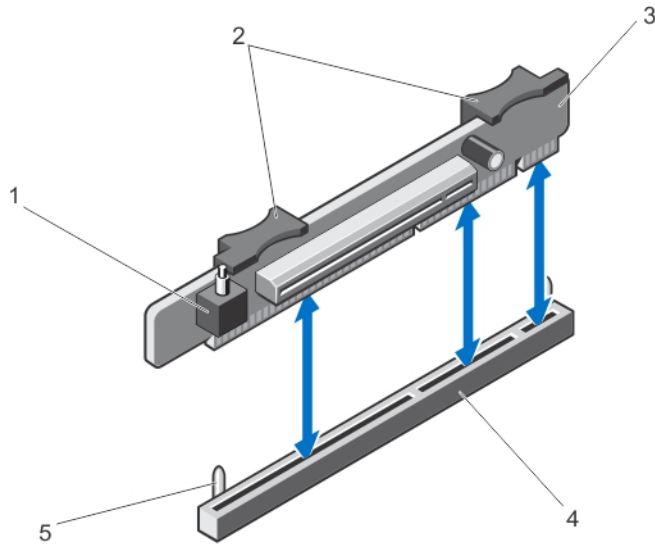
그림 33. 확장 카드 라이저 2 분리 및 설치
