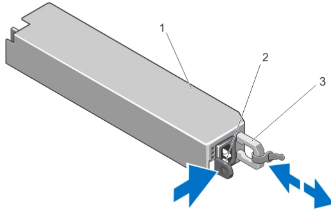
그림 40. 중복 전원 공급 장치 분리 및 설치
