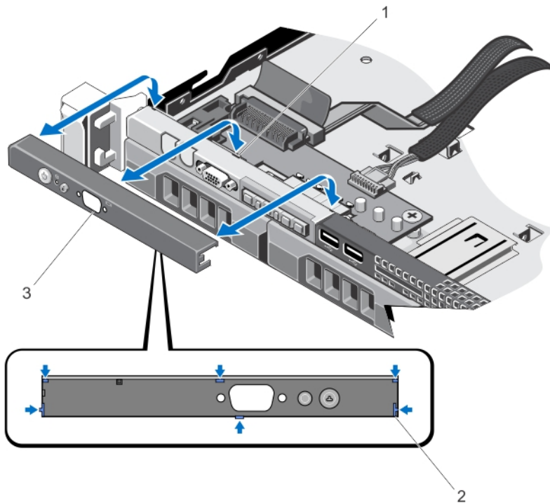
그림 52. 제어판 분리 및 설치—4개 하드 드라이브 시스템
