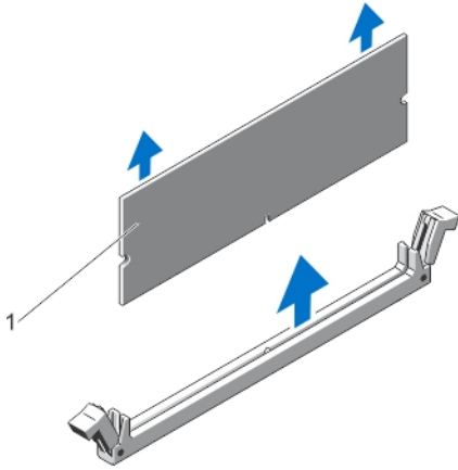
그림 16. 메모리 모듈 분리
