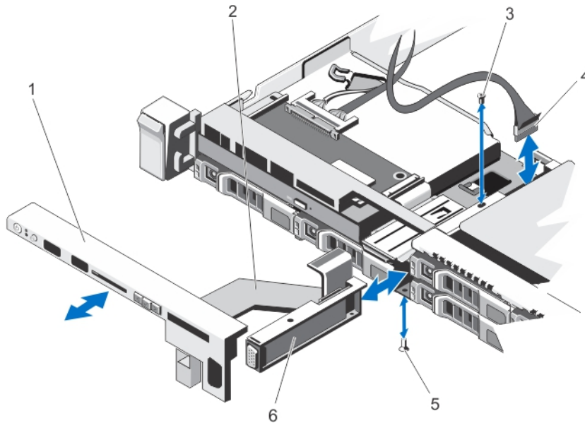
그림 57. VGA 모듈 분리 및 설치
