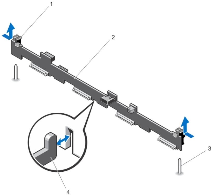
그림 46. 4개 하드 드라이브 후면판 분리 및 설치
