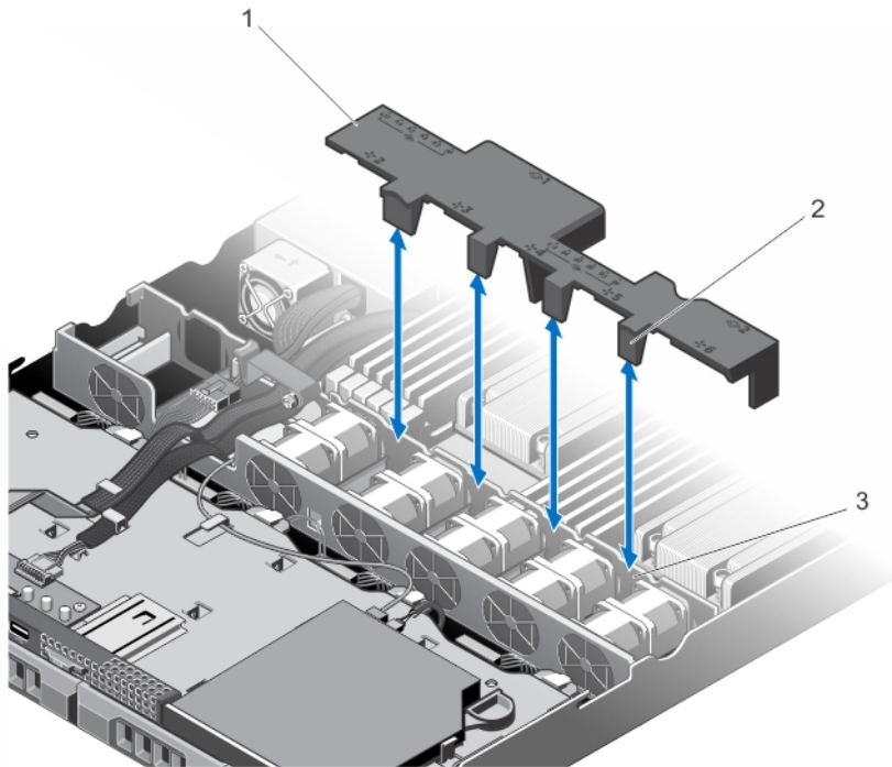
그림 13. 냉각 덮개 분리 및 설치
