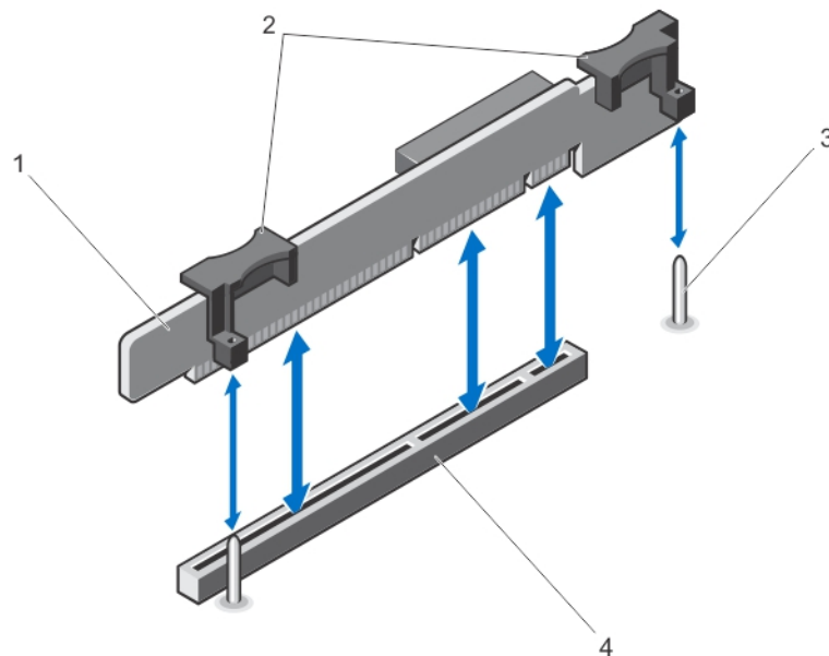
그림 32. 확장 카드 라이저 1 분리 및 설치
