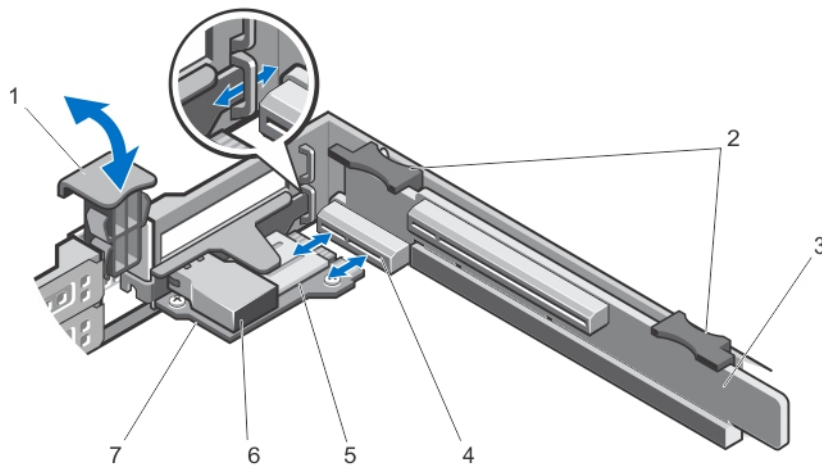
그림 34. iDRAC Ports 카드 분리 및 설치
