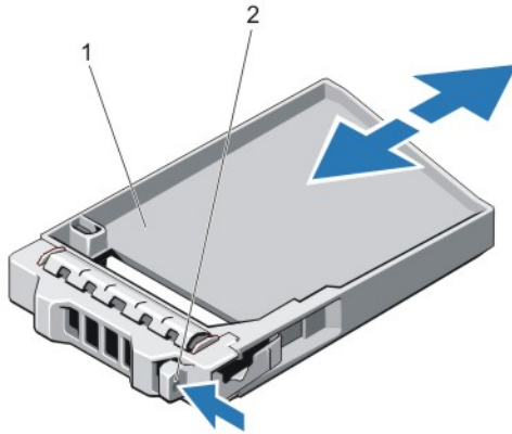
그림 18. 2.5인치 하드 드라이브 보호물 분리 및 설치
