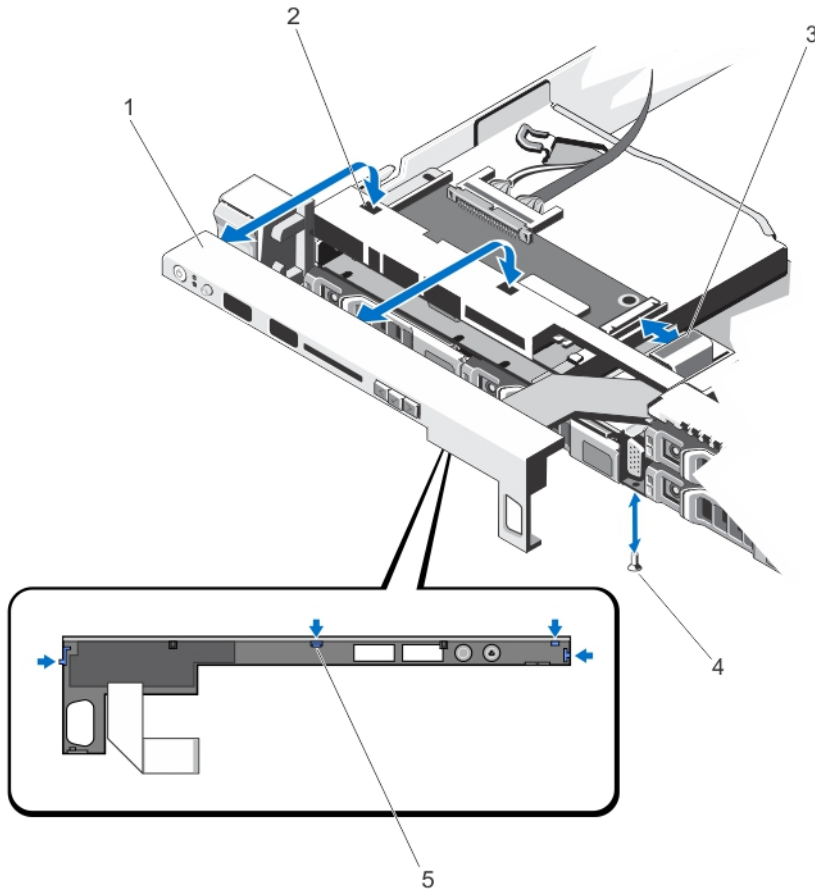
그림 53. 제어판 분리 및 설치—8개 하드 드라이브 시스템
