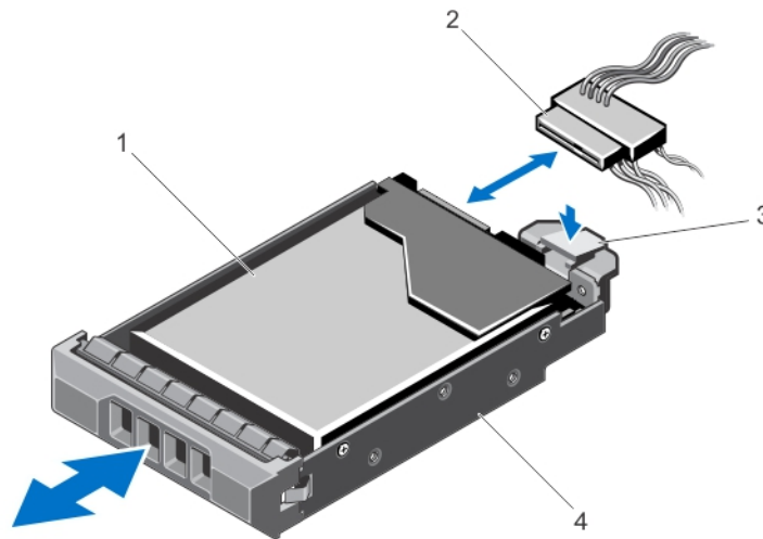
그림 21. 케이블 연결된 하드 드라이브 분리 및 설치
