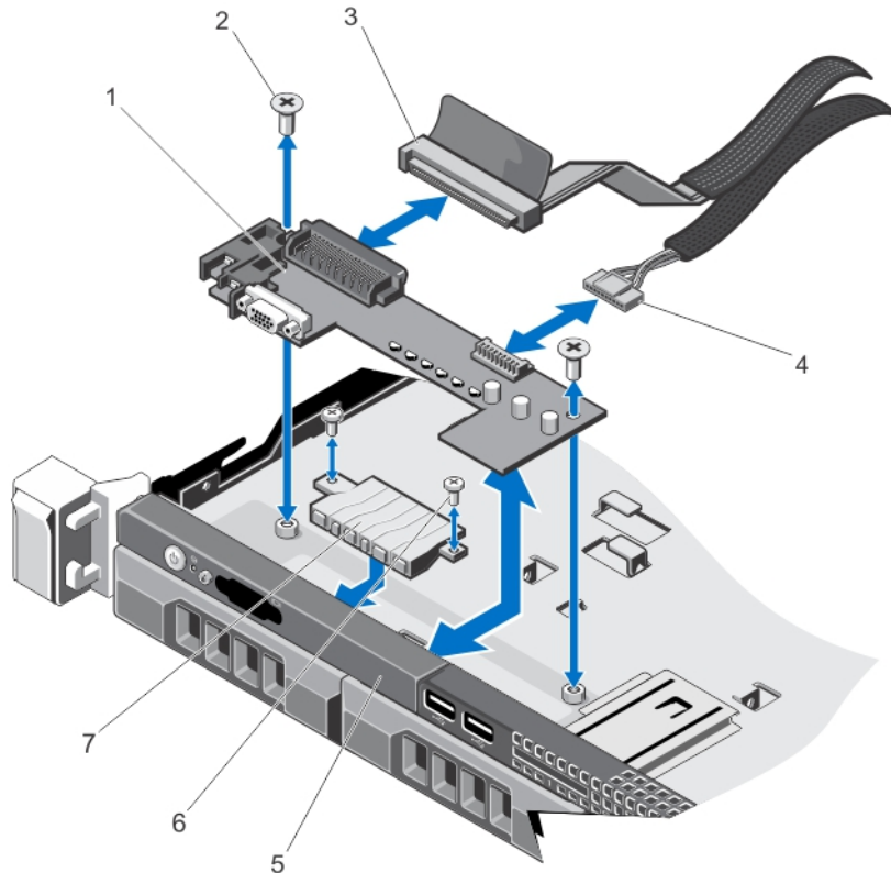
그림 54. 제어판 모듈 분리 및 설치—케이블 연결된 3.5인치 하드 드라이브 시스템
