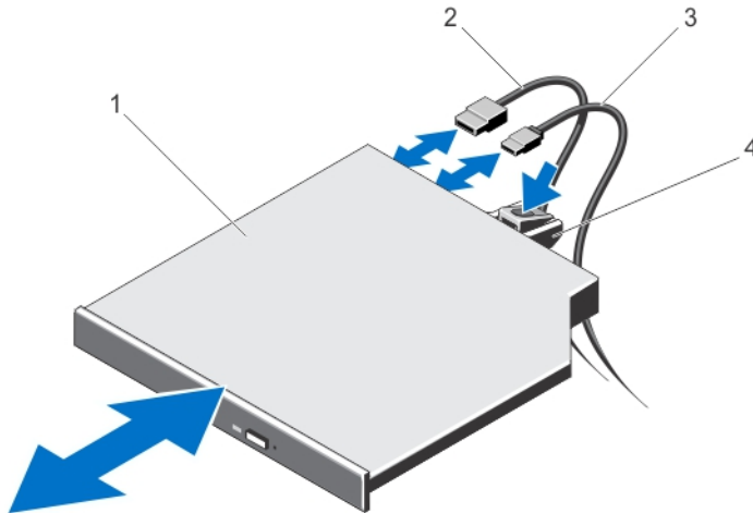
그림 26. 광학 드라이브 분리 및 설치(핫 스왑 가능한 하드 드라이브 시스템)
