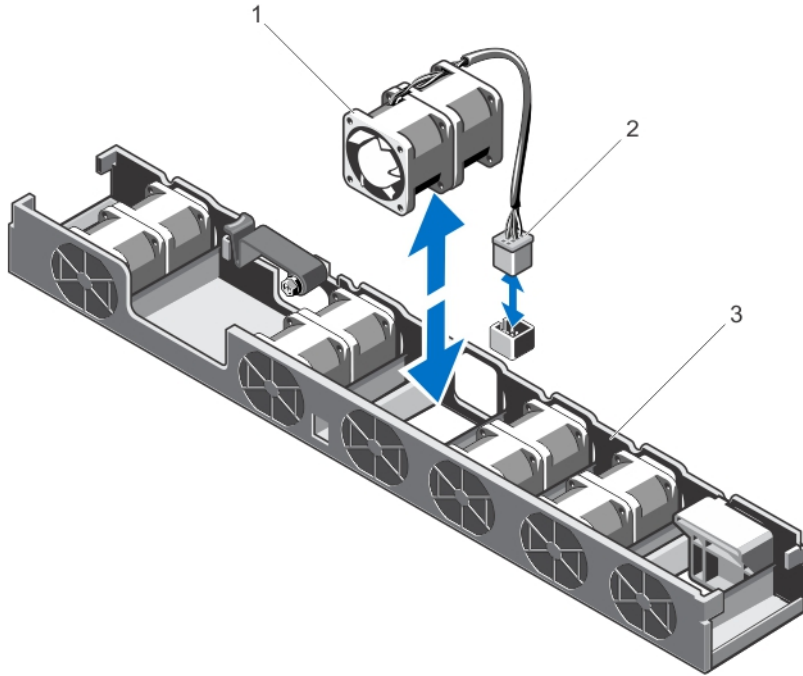
그림 28. 냉각 팬 분리 및 설치
