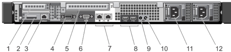
그림 6. 후면 패널 구조 및 표시등
