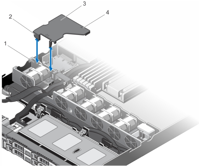
그림 58. PDB 덮개 분리 및 설치
