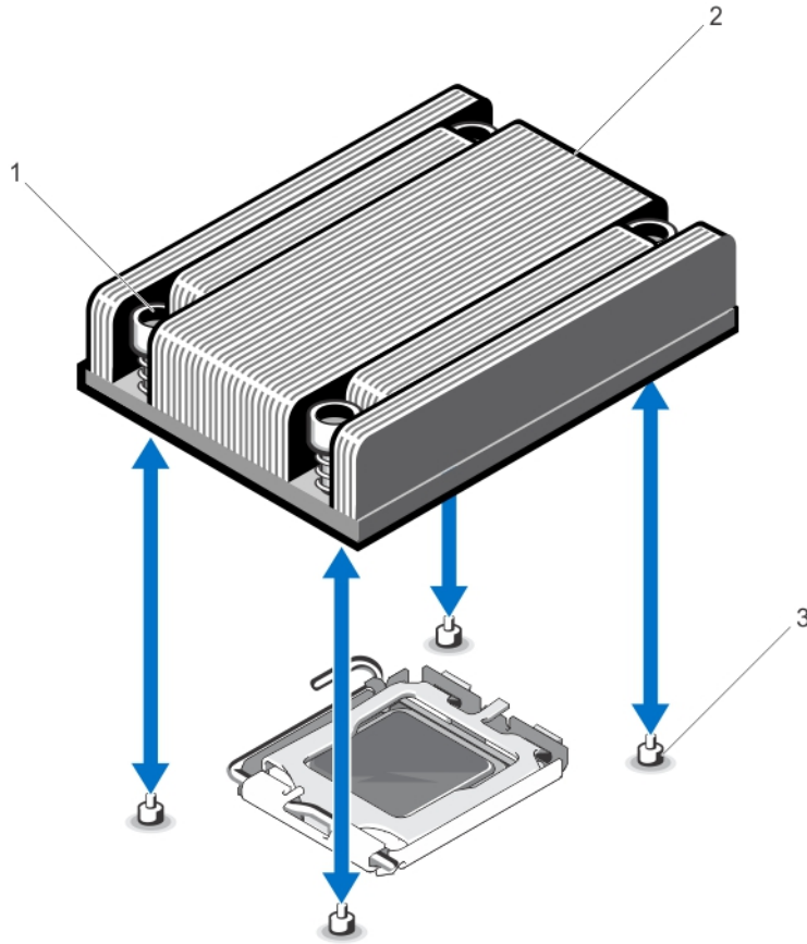
그림 38. 프로세서 방열판 분리 및 설치
