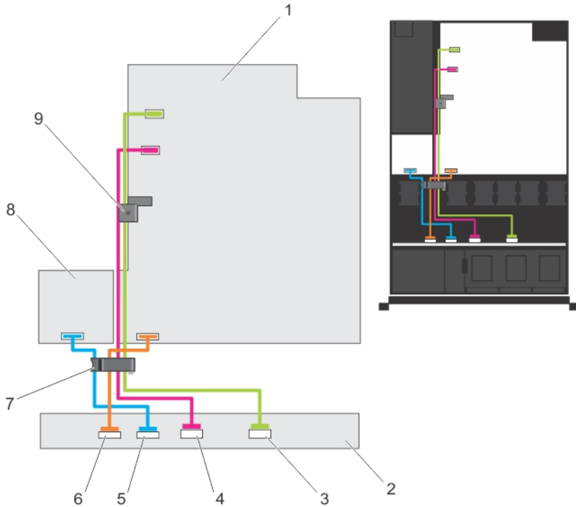
그림 51. 케이블 연결 다이어그램—8개 하드 드라이브 후면판
